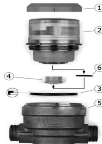
Flaches UP-Gehäuse MO-C
